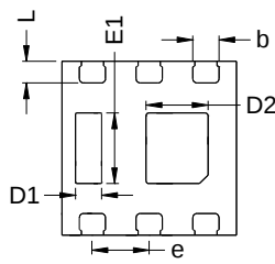
Bottom View 背面视图
