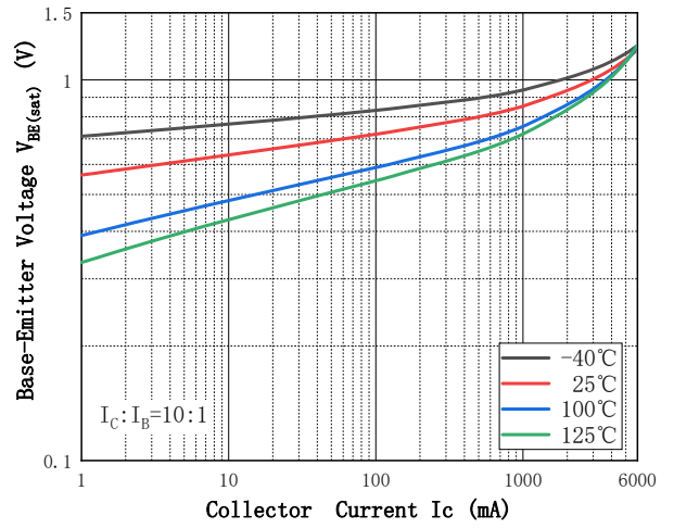
Fig.4 - Base-Emmitter Voltage
